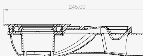
SECCIÓN A-A
