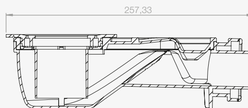
SECCIÓN B-B
