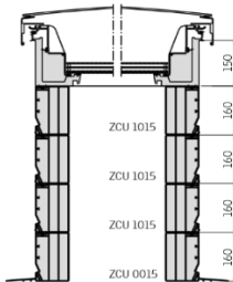
Ventana de cubierta plana CVU/CFU con juego de casetones ZCU S000 con juego de casetones ZCU 0015 y ZCU 1015 y un adaptador de casetón ZCU 0015 y ZCU 1015. Se pueden apilar hasta tres adaptadores de casetón ZCU 1015. Altura máxima: 790 mm
