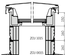
Ventana de cubierta plana CVU/CFU Con casetones ZCU 0015 y ZCU 1015
