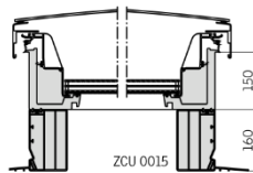
Ventana de cubierta plana CVU/CFU con un montantes ZCU 0015
